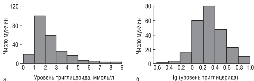
Рис. 8.3. Логнормальное распределение уровня триглицерида у 232 мужчин с заболеваниями сердца (глава 19) (а). Почти нормальное распределение \log_{10} (уровень триглицерида) (б)
