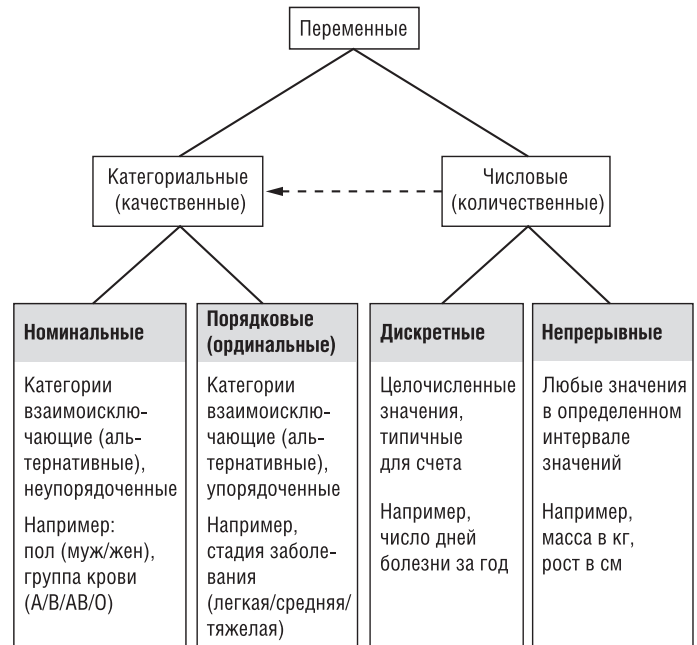
Рис. 1.1. Схема, показывающая различные типы переменных
