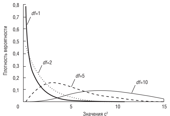
Рис. 8.2. \chi^2 распределения Пирсона со степенями свободы ( df )=1, 2, 5 и 10
