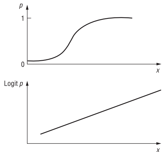
Рис. 9.3. Эффект логистического преобразования сигмовидной кривой
