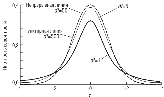
Рис. 8.1. t -распределение со степенями свободы ( df )=1; 5; 50 и 500
