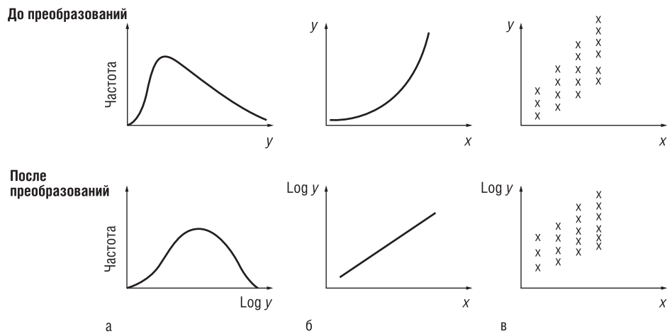
Рис. 9.1. Свойства логарифмического преобразования: нормализация (а), линейзация (б), выравнивание дисперсий (в)
