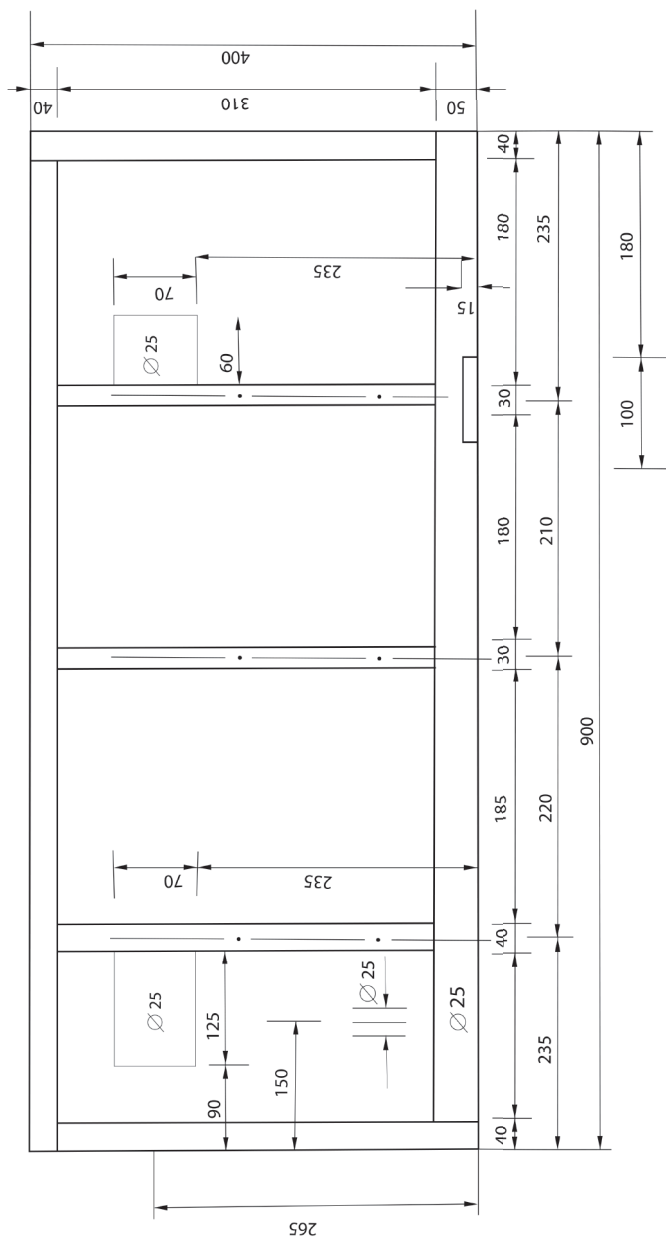
Схема корпуса улья № 2. Все измерения указаны в миллиметрах
