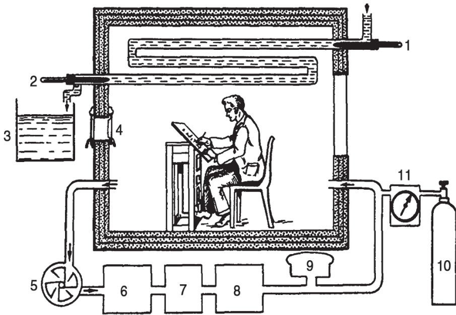
Рис. 1.1. Прямая калориметрия (биокалориметр Этютера-Бенедикта): 1-3 — жидкостный теплообменник; 4 — окно для наблюдения; 5 — вентилятор; 6-7 — фильтры; 8 — поглотитель влаги; 9 — поглотитель CO 2 ; 10-11 — баллон с кислородом и манометром
