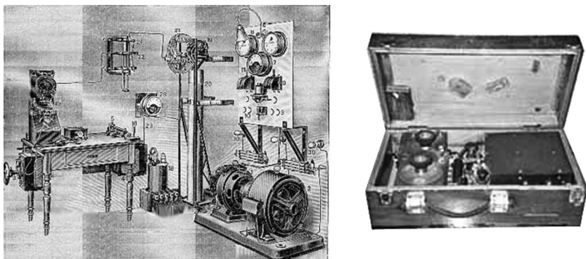
Рис. 2.11. Общий вид искровых стационарной (слева) и портативной радиостанций РОБТиГ [4]
